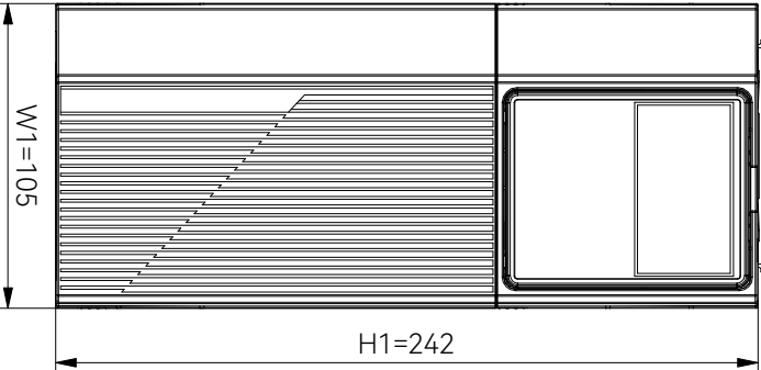
主视图
