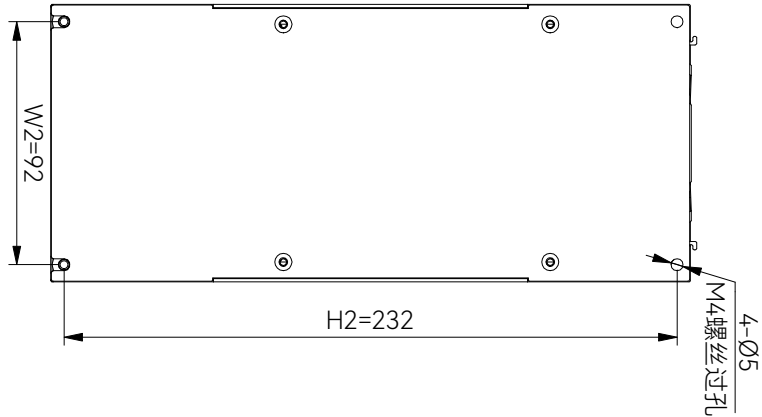
后视图
