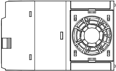
主视图
