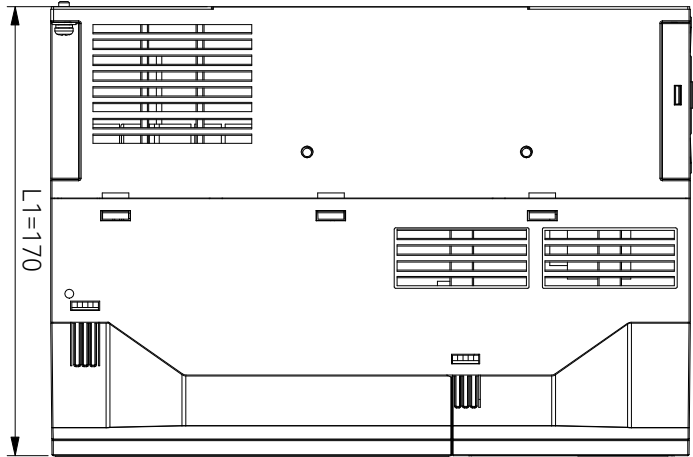
右视图
