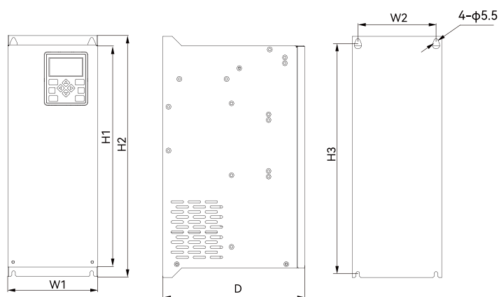
图 1-4 E630 30~45kW 系列尺寸示意图
