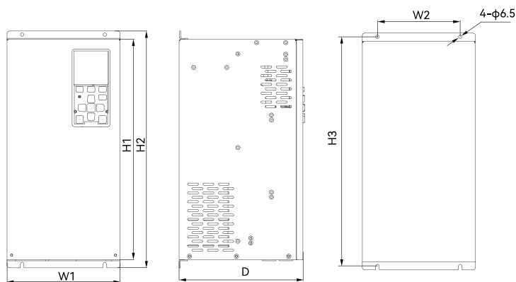
图 1-5 E630 75kW 系列尺寸示意图
