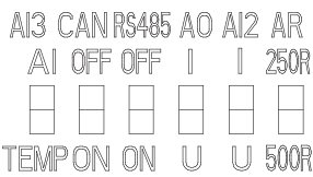
图 1-3 拨码开关示意图
