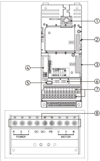
图 1-2 E630 系列接口示意图
