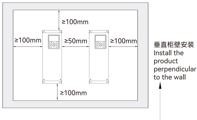
图 3-1 E630 控制柜安装示意图
