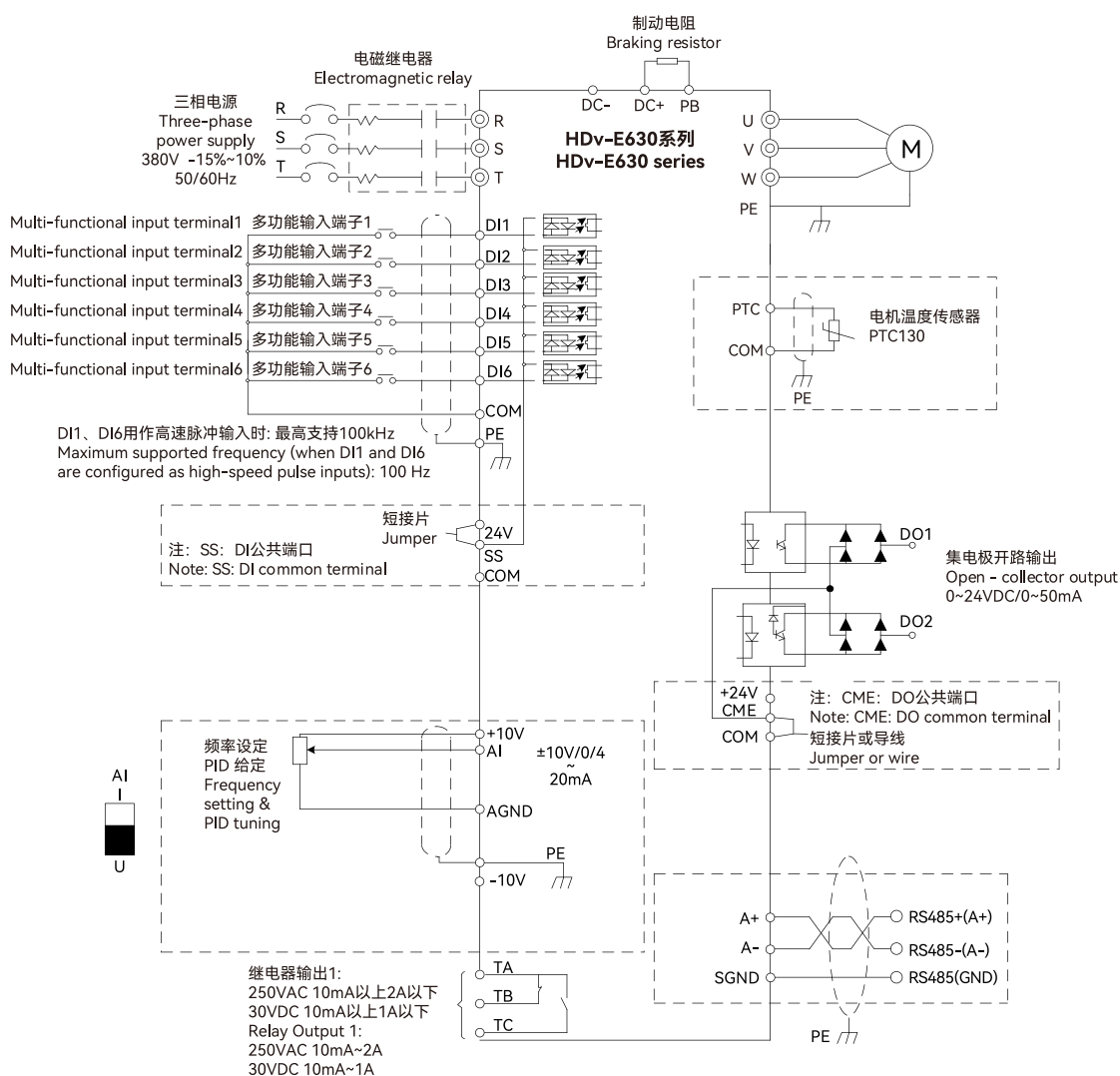
图 3-3 HDv-E630 系列三相 380V 机种标准接线
