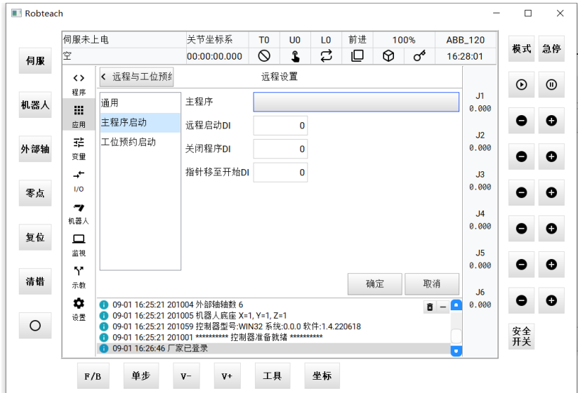
图12-3 主程序启动界面示意图
