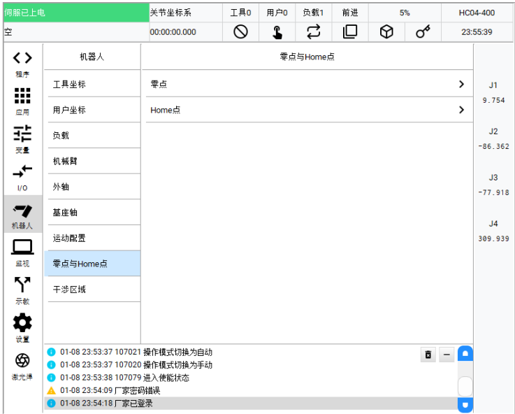
图7-8-1 零点和Home点界面图
