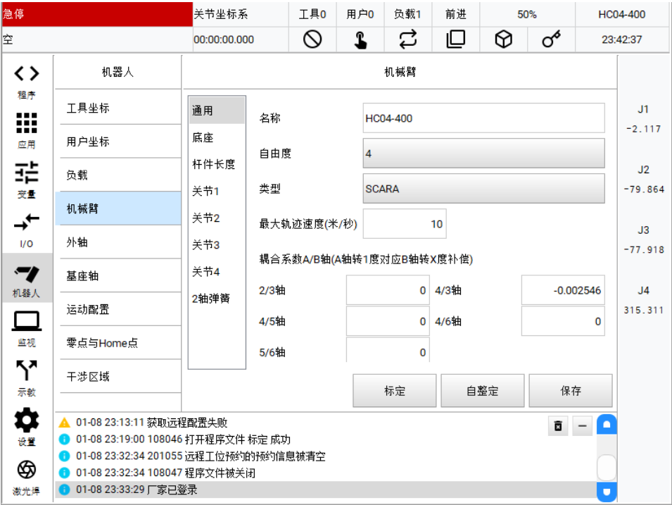
图7-4-1 机械臂界面参数图
