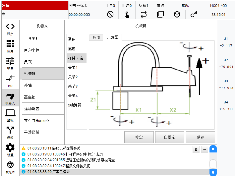
图7-4-5 4轴SCARA机器人杆件长度示意图
