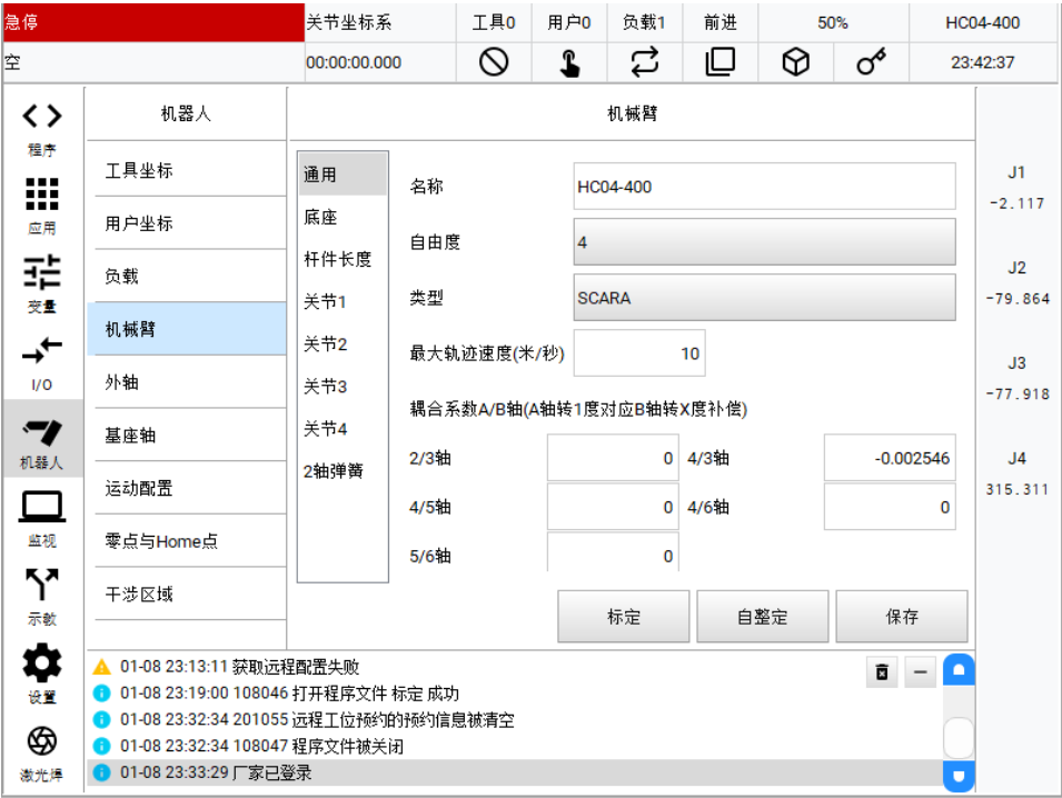
图7-4-2 通用设置界面参数图
