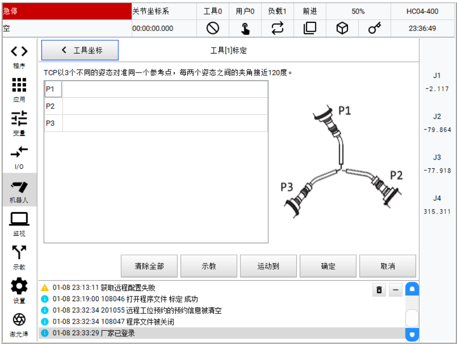
图7-1-4 3点法标定界面示意图
