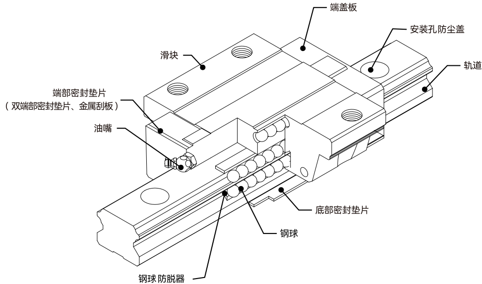
【HBH导轨结构示意图】
