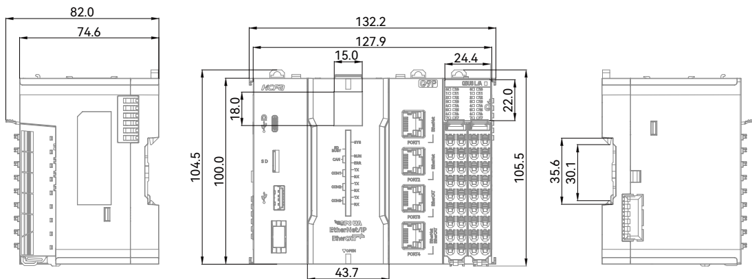
图 9 HCQ9P 安装尺寸 (单位: mm)
