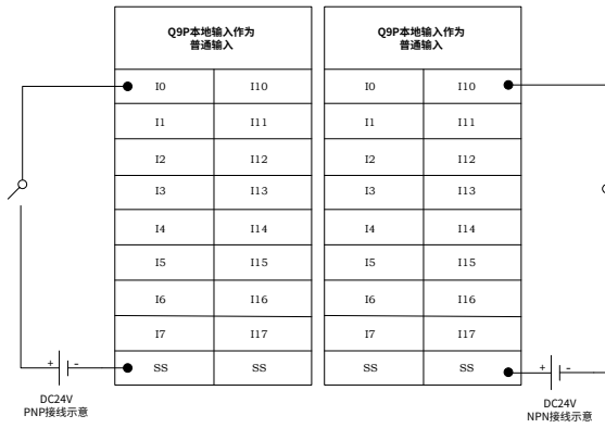
图 15 本地输入作为普通输入外部接线图
