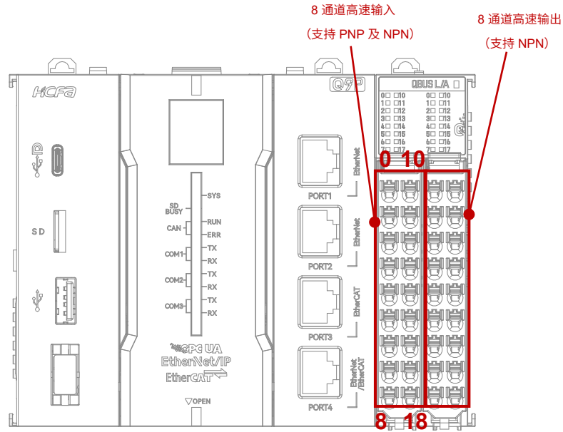
图 10 HCQ9P CPU 模块 IO 通道示意图
