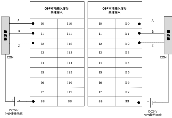
图 16 本地输入作为高速输入外部接线图
