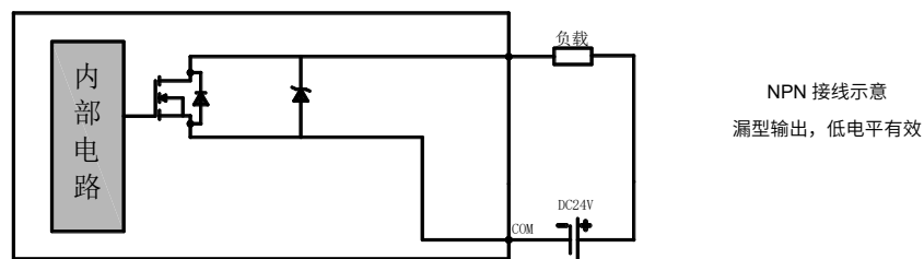
图 14 本地输出作为高速输出内部电路简图
