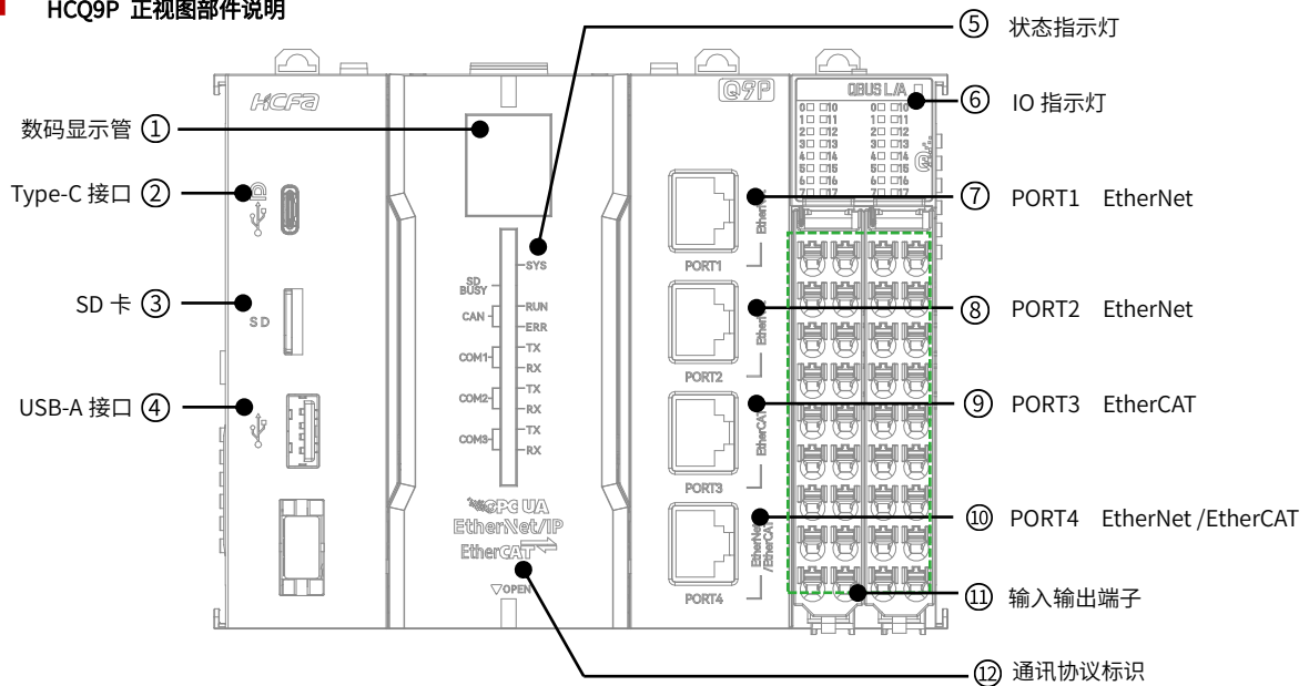
图 2 HCQ9P 正视图部件说明图
