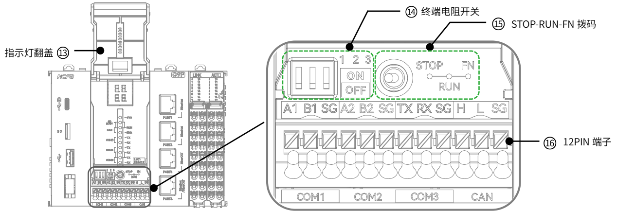
图 3 HCQ9P 正视图翻盖端子说明图
