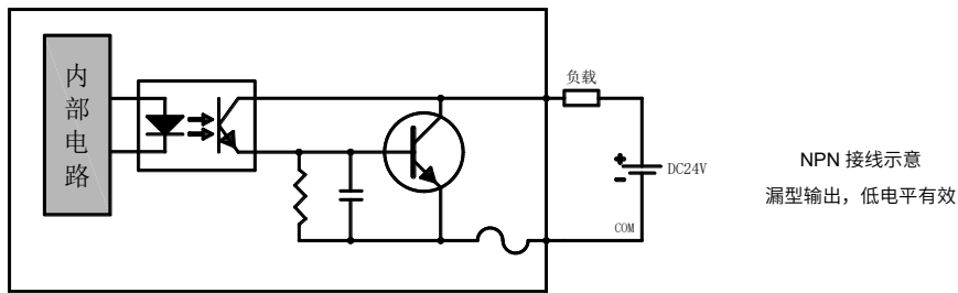
图 13 本地输出作为普通输出内部电路简图
