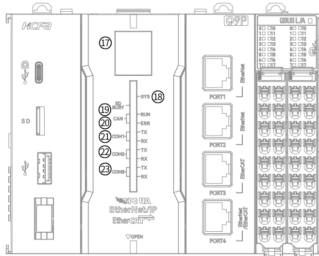
图4 HCQ9P 状态指示灯说明图
