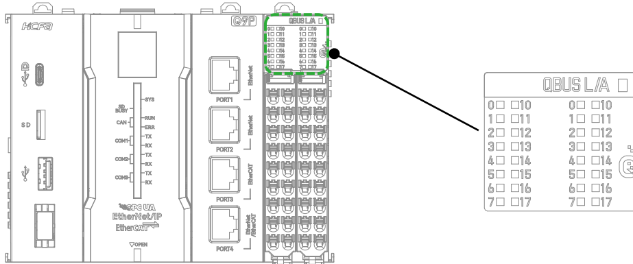
图 5 HCQ9P IO 端子及 IO 灯板说明图
