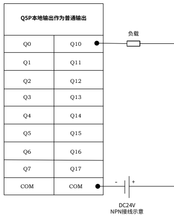
图 17 本地输出作为普通输出外部接线图
