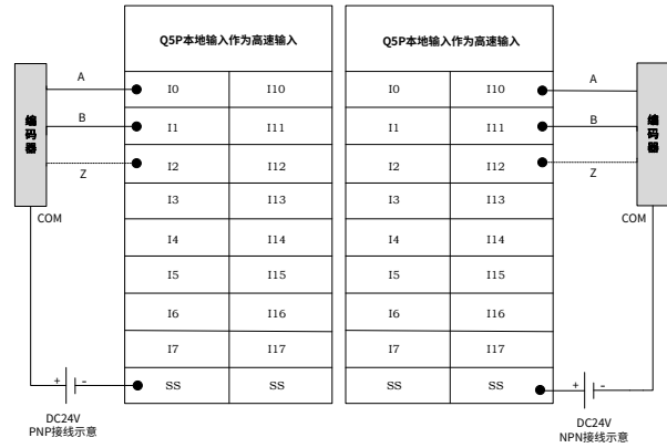
图 16 本地输入作为高速输入外部接线图
