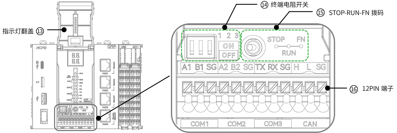
图 3 HCQ5P 正视图翻盖端子说明图
