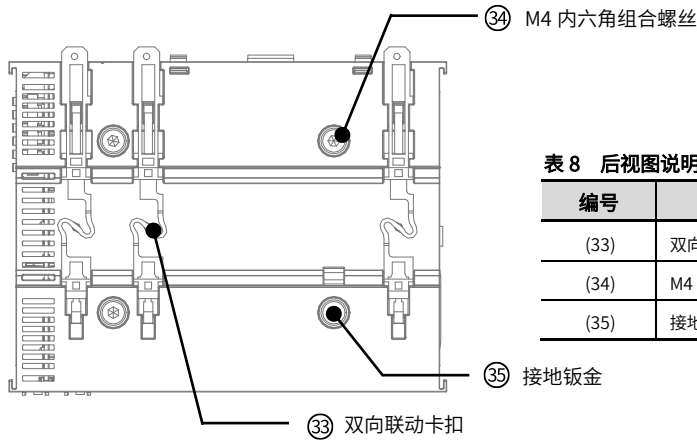
图8 HCQ5P 后视图说明图
