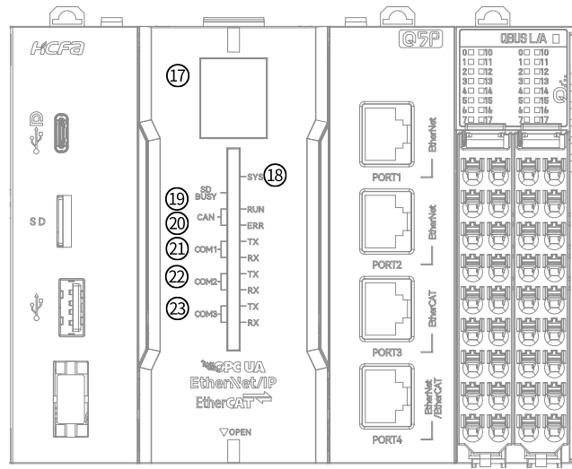
图4 HCQ5P 状态指示灯说明图
