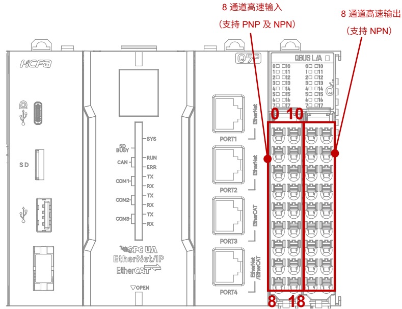
图 10 HCQ5P CPU 模块 IO 通道示意图
