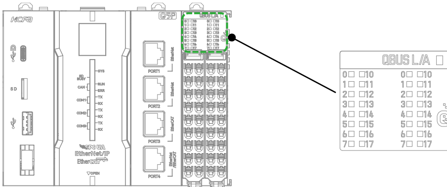
图 5 HCQ5P IO 端子及 IO 灯板说明图
