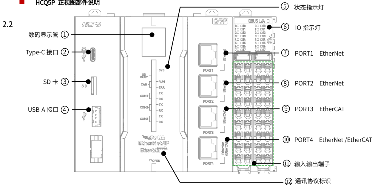
图 2 HCQ5P 正视图部件说明图
