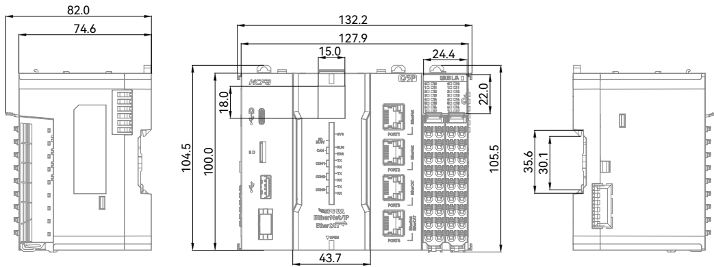
图9 HCQ5P 安装尺寸 (单位: mm)
