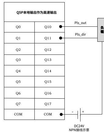
图 18 本地输出作为高速输出外部接线图
