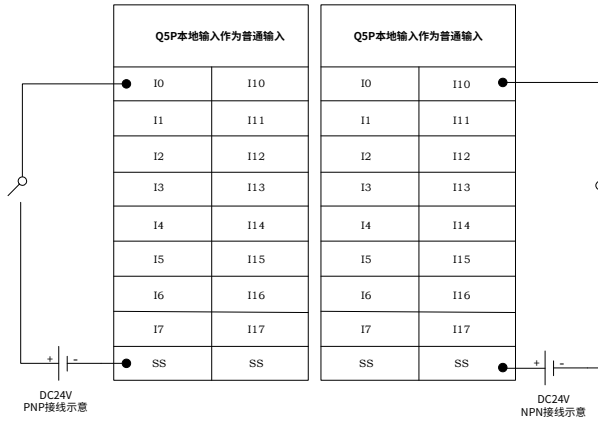
图 15 本地输入作为普通输入外部接线图
