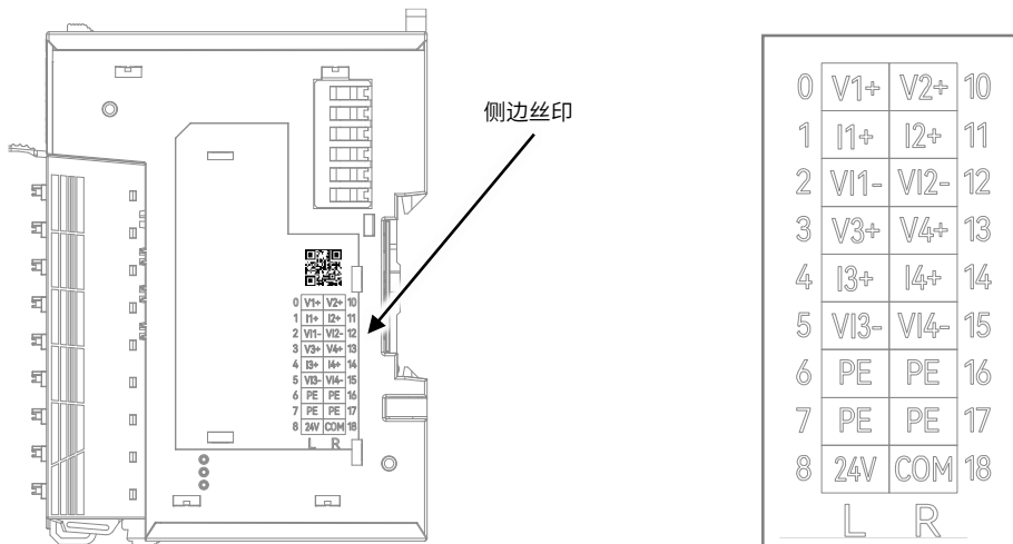
图 4 HCMX-DA04-D 模块侧边丝印
