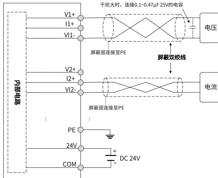
图 6 HCMX-DA04-D 模块内部接线图
