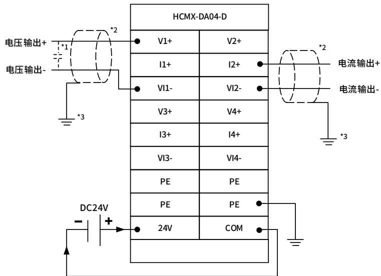
图 7 HCMX-DA04-D 模块端子接线图
