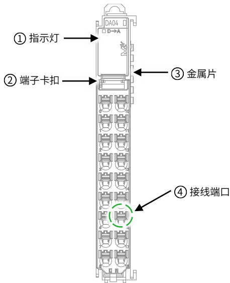
图 2 HCMX-DA04-D 正视图部件图
