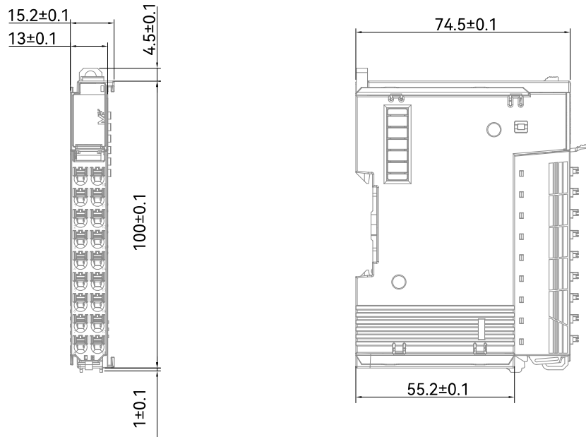
图5 HCMX-DA04-D 模块尺寸图
