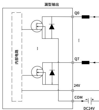
图 9 本地输出内部电路简图
