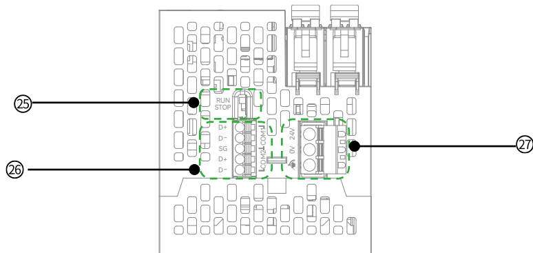
图 5 HCM511S CPU 单元俯视图说明图
