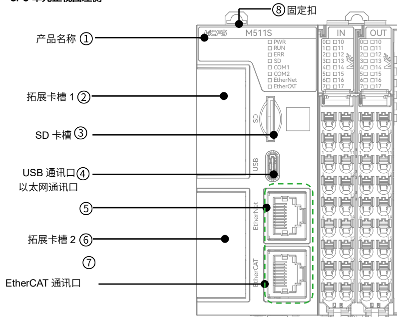
图 2 HCM511S CPU 单元正视图左侧说明图
