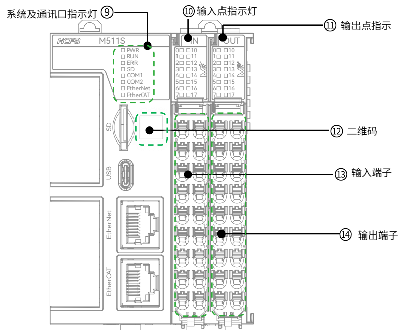
图 3 HCM511S CPU 单元正视图右侧说明图
