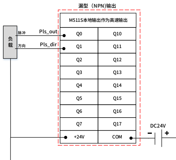
图 13 本地输出作为高速输出外部接线图
