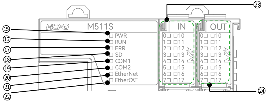
图 4 HCM511S CPU 单元指示灯说明图
