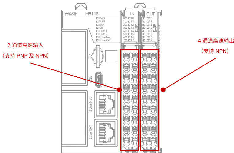
图 7 M511S CPU 模块 IO 通道示意图
