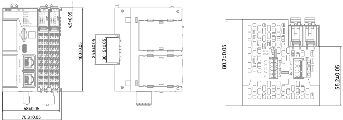
图 6 HCM511S 控制器主机安装尺寸 (单位: mm)
