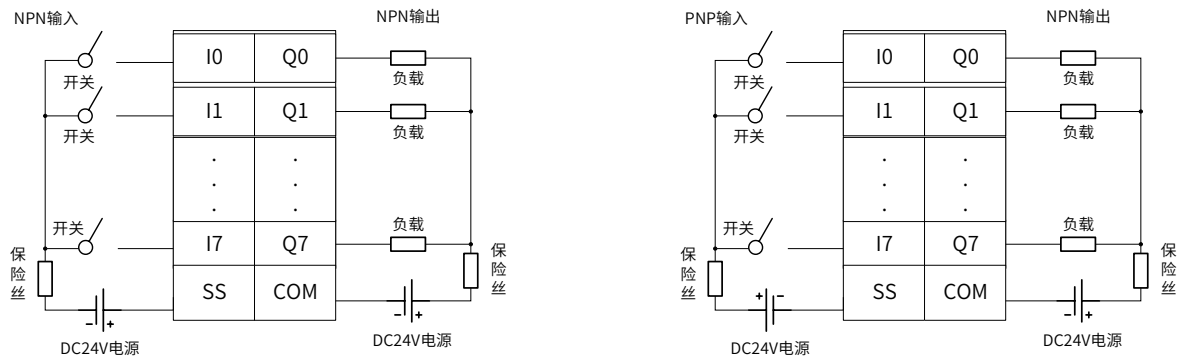
图 28 数字量混合模块 HCQX-MD16/32-D4 端子接线电路图
