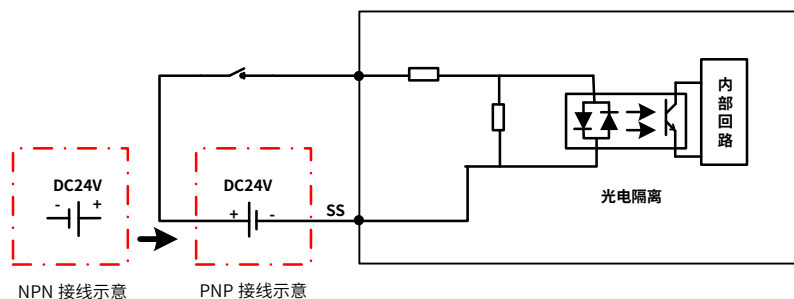
图 22 数字量输入模块 HCQX-ID16/32-D4 内部电路图
