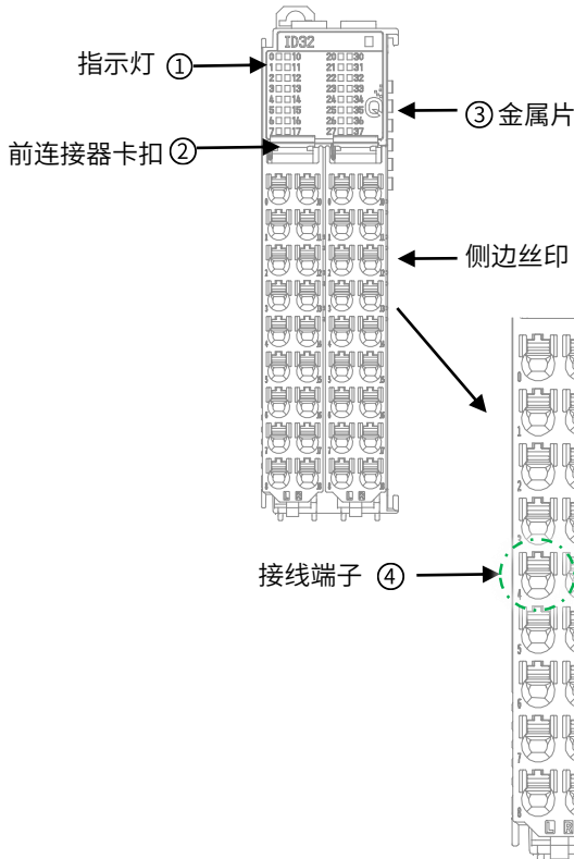
图 5 HCQX-ID32-D4 接口示意图
