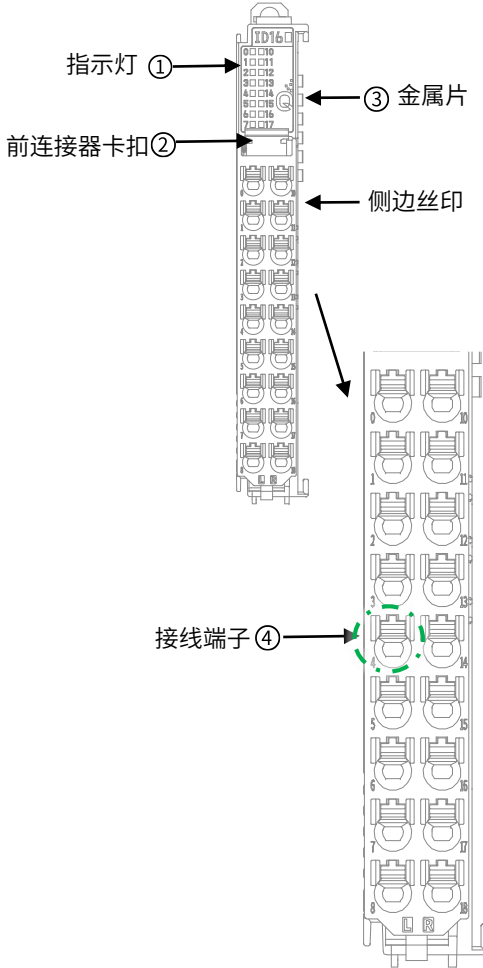
图2 HCQX-ID16-D4 接口示意图
