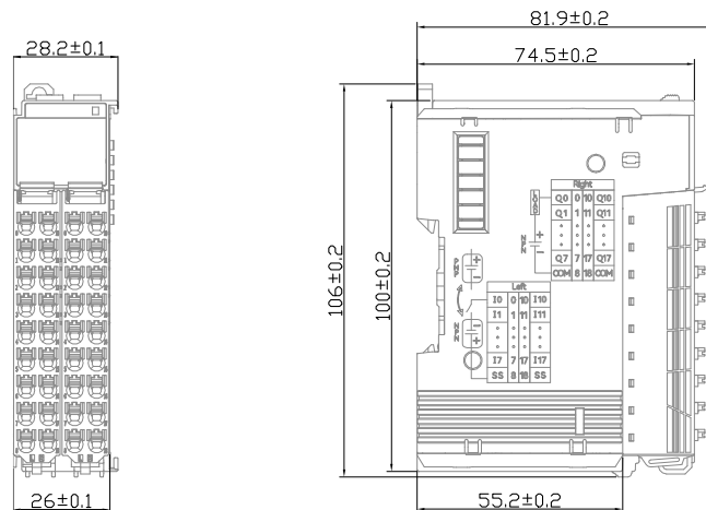
图 21 HCQX-ID/OD/MD32-D4 扩展模块安装尺寸 (单位: mm)
