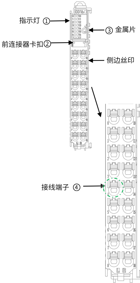
图 8 HCQX-OD16-D4 接口示意图
