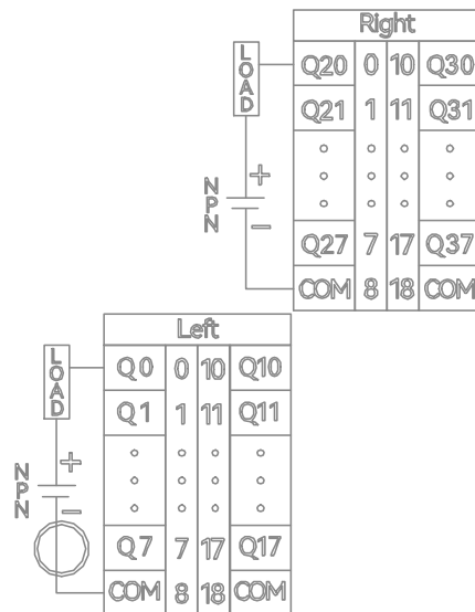
图 12 HCQX-OD32-D4 侧边丝印图
