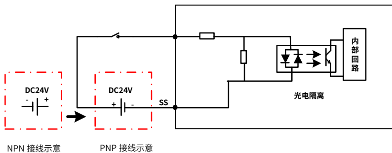
图 26 数字量混合模块 HCQX-MD16/32-D4 输入部分内部电路图
