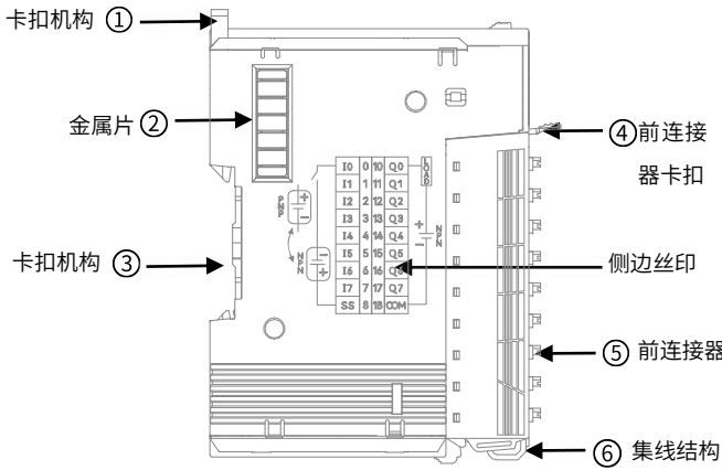
图 20 数字量模块侧视图
