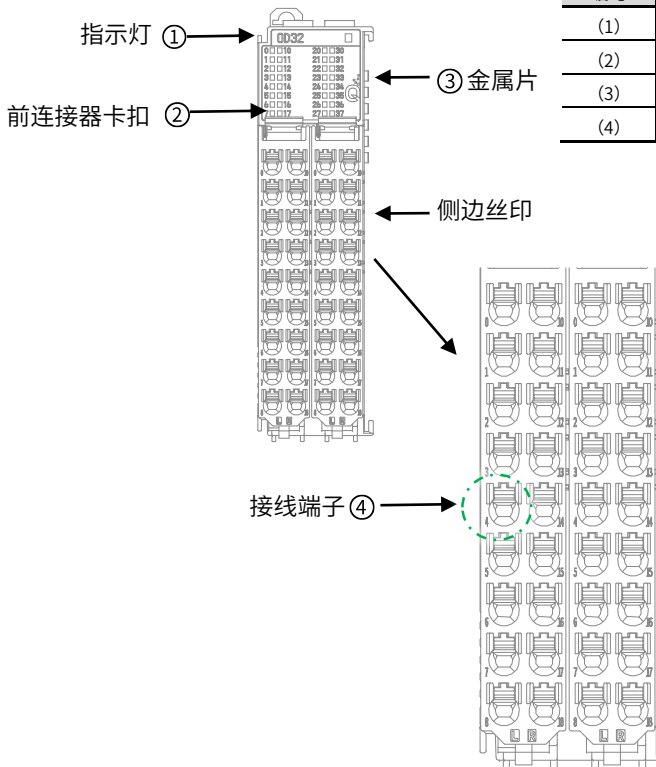
图 11 HCQX-OD32-D4 接口示意图
