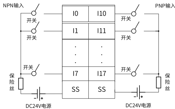
图 23 数字量输入模块 HCQX-ID16/32-D4 端子接线图
