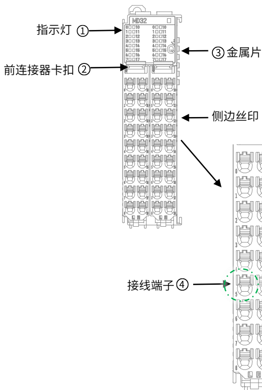
图 17 HCQX-MD32-D4 接口示意图
