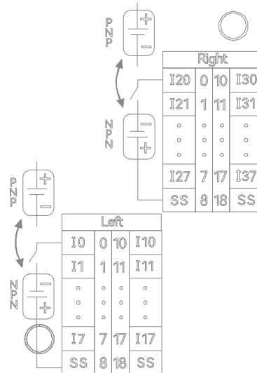
图 6 HCQX-ID32-D4 侧边丝印图
