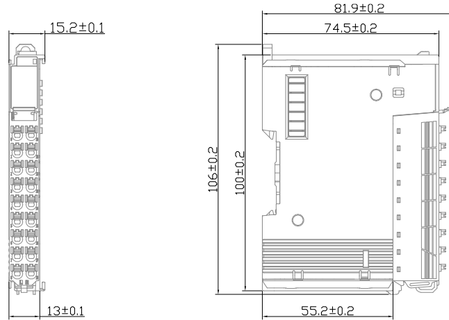
图 20 HCQX-ID/OD/MD16-D4 扩展模块安装尺寸 (单位: mm)
