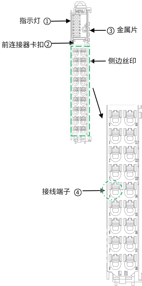
图 14 HCQX-MD16-D4 接口示意图
