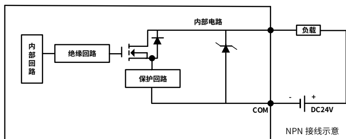
图 24 数字量输出模块 HCQX-OD16/32-D4 内部电路图
