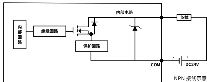
图 27 数字量混合模块 HCQX-MD16/32-D4 输出部分内部电路图
