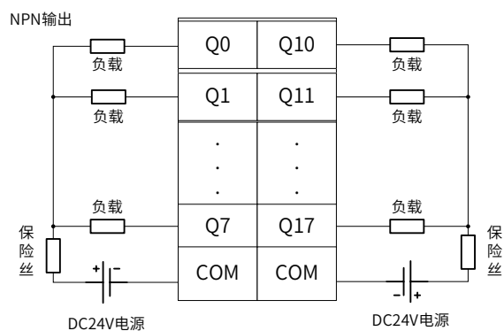
图 25 数字量输出模块 HCQX-OD16/32-D4 端子连接图
