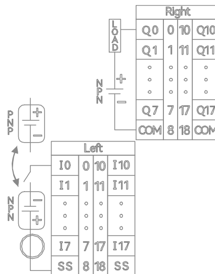
图 18 HCQX-MD32-D4 侧边丝印图
