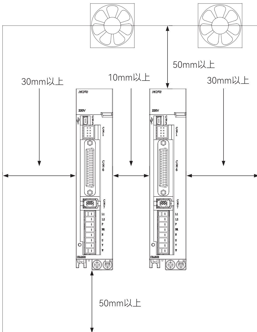
驱动器的安装间隔图
