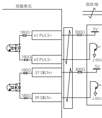
NPN型
