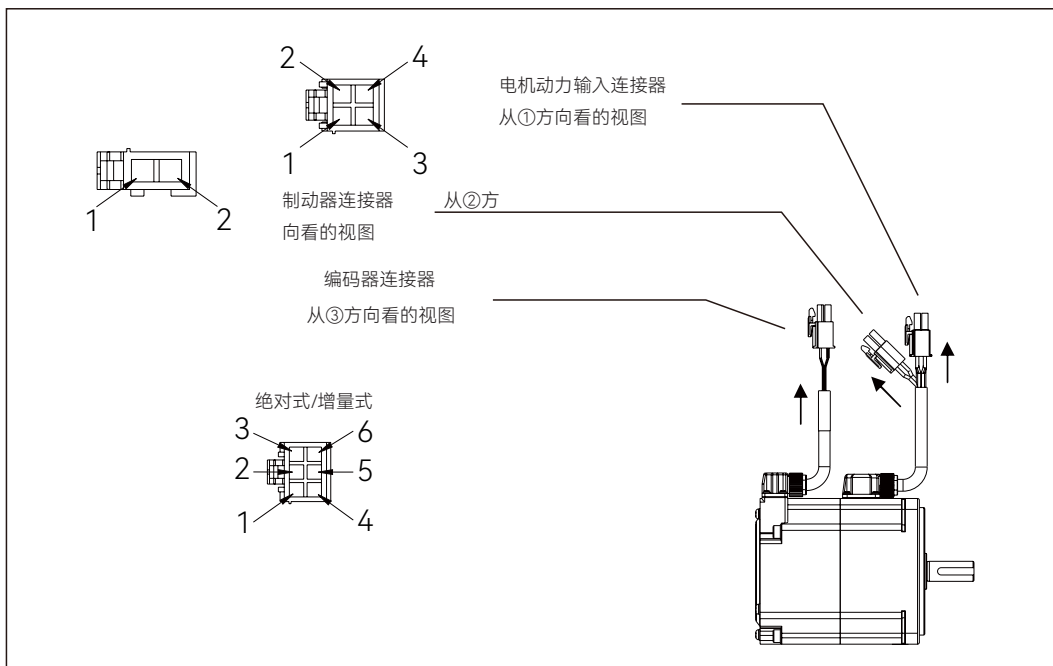
电机连接器和插针排列 (50~750W)
