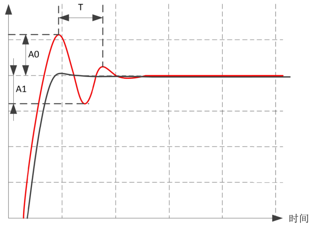
定位控制时低频振动波形
