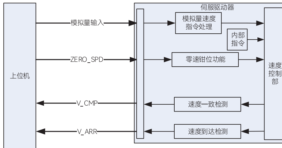
速度控制基本功能框图
