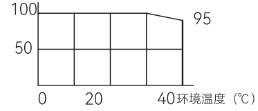
连续转矩-环境温度
