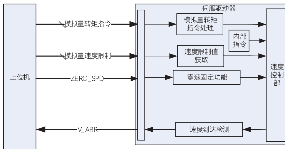
转矩控制基本功能框图
