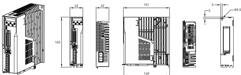
驱动器200W及以下
