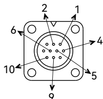
绝对式/增量式编码器连接器
