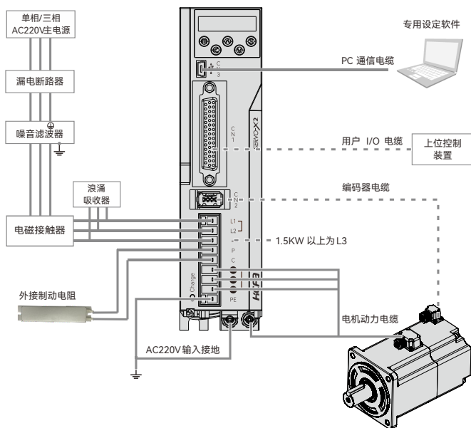
图4.1.1 系统配线图
