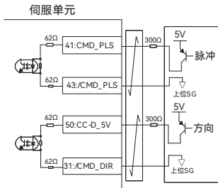
5V集电极PNP型
