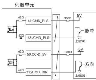
5V集电极NPN型
